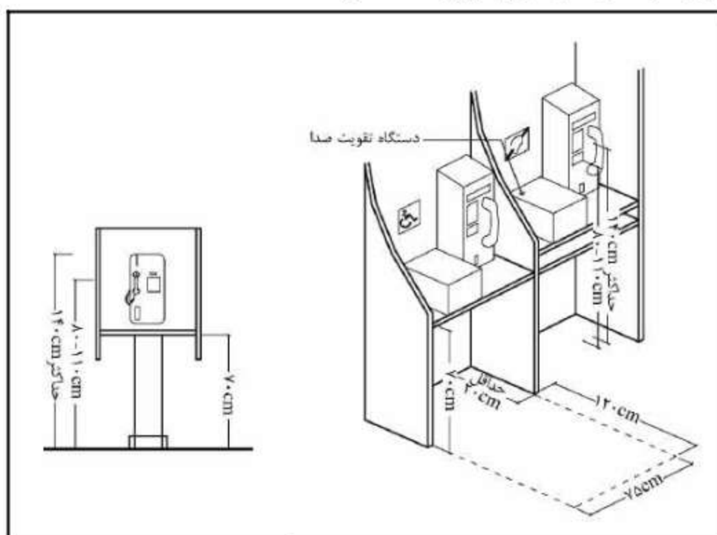
شکل ۲-۳۳- تلفن عمومی دسترس‌پذیر
