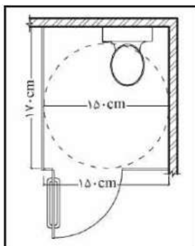
شکل ۳-۲۸- حداقل ابعاد فضای سرویس بهداشتی
