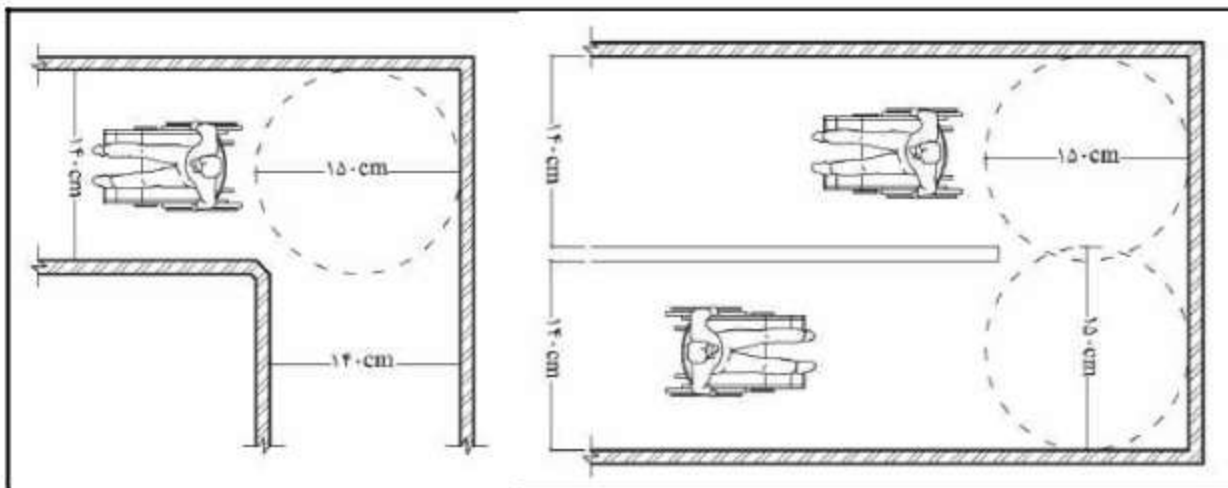
شکل ۳-۳- تامین فضا برای امکان چرخش ۹۰ و ۱۸۰ درجه‌ای
