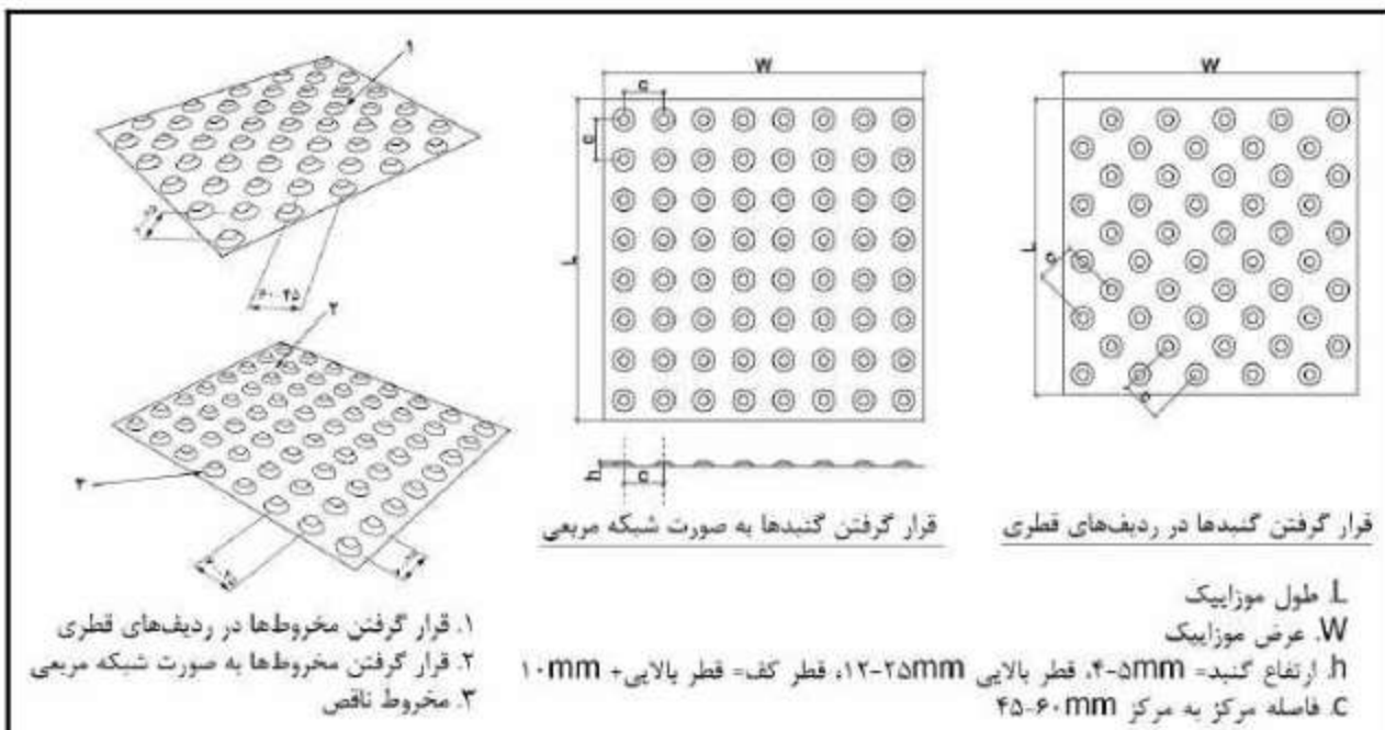
شکل ۲-۹- چیدمان، فواصل و ابعاد کفیوش سکه‌ای
