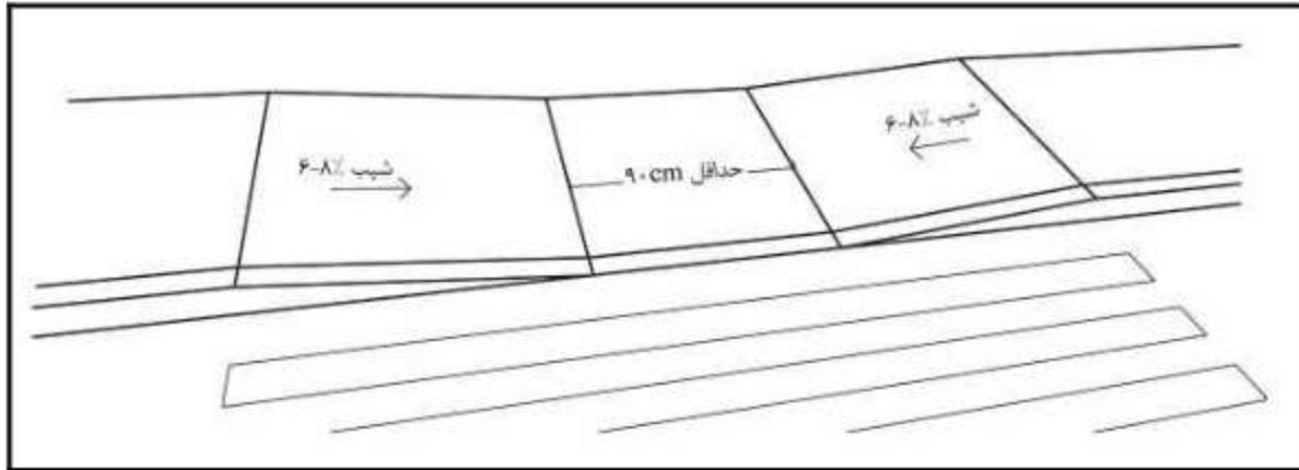
شکل ۲-۱۸- رمپ جدول موازی
