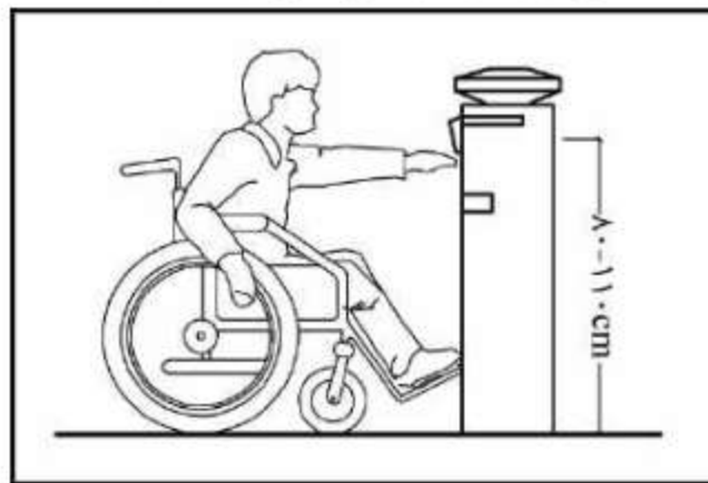
شکل ۲-۳۶- ارتفاع شکاف صندوق پست دسترس پذیر
