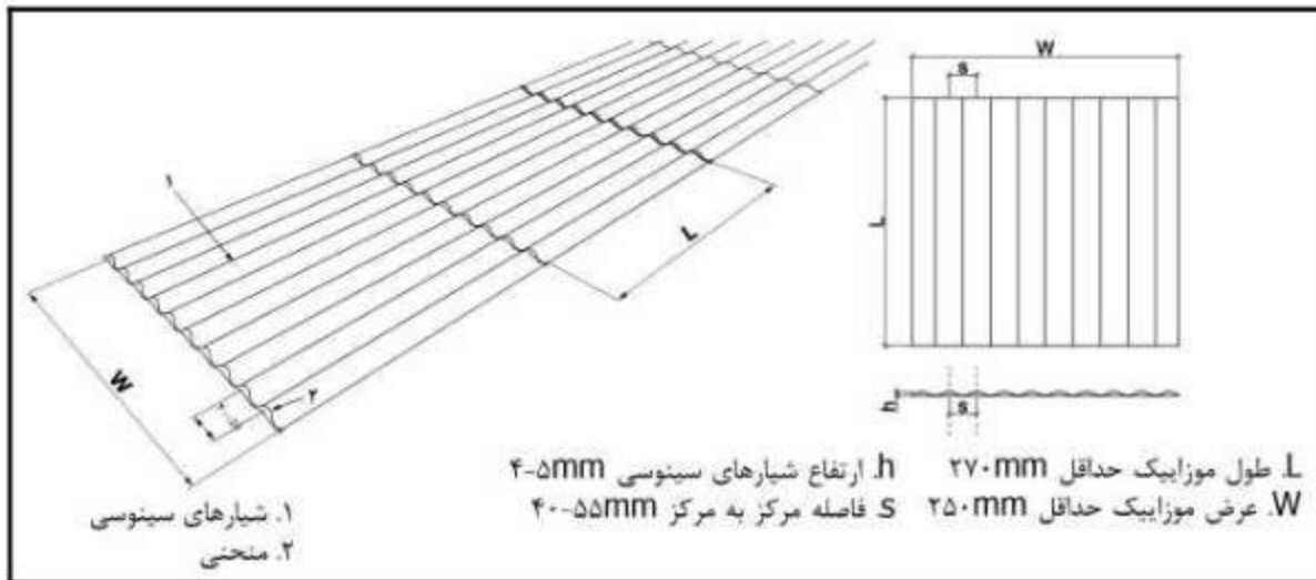
شکل ۲-۸- چیدمان، فواصل و ابعاد کفیوش شیاردار سینوسی
