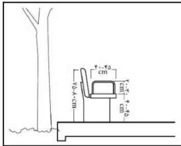
شکل ۲-۳۱- ابعاد نیمکت
