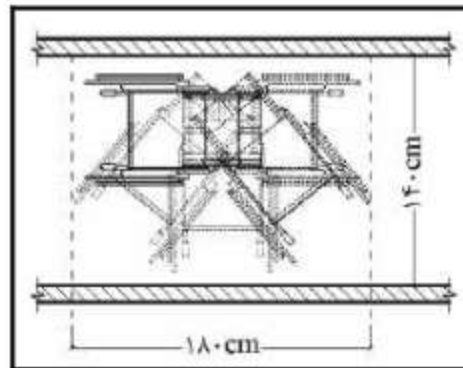
شکل ۷-۱- سطح موردنیاز برای گردش ۱۸۰ درجه‌ای صندلی چرخدار
