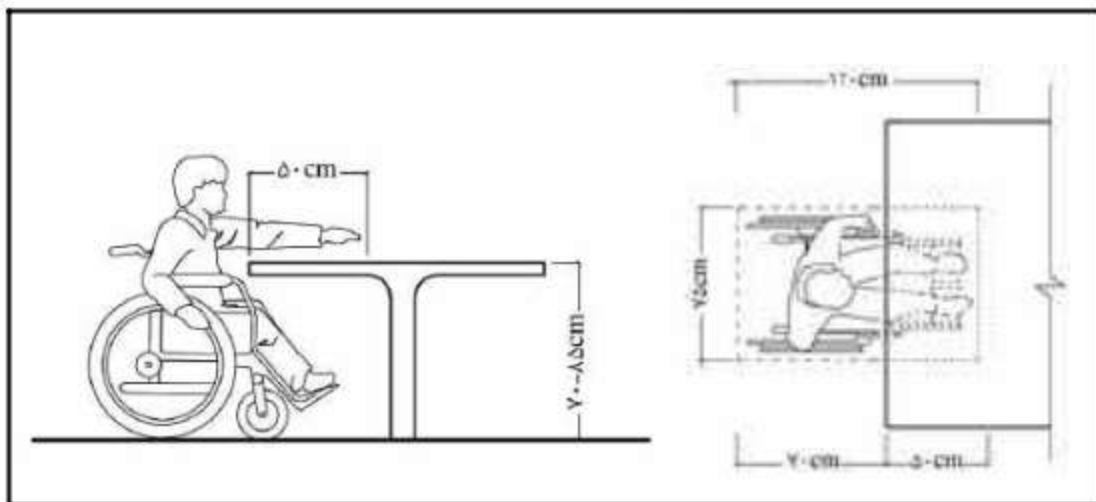
شکل ۲-۳۲- ابعاد میز
