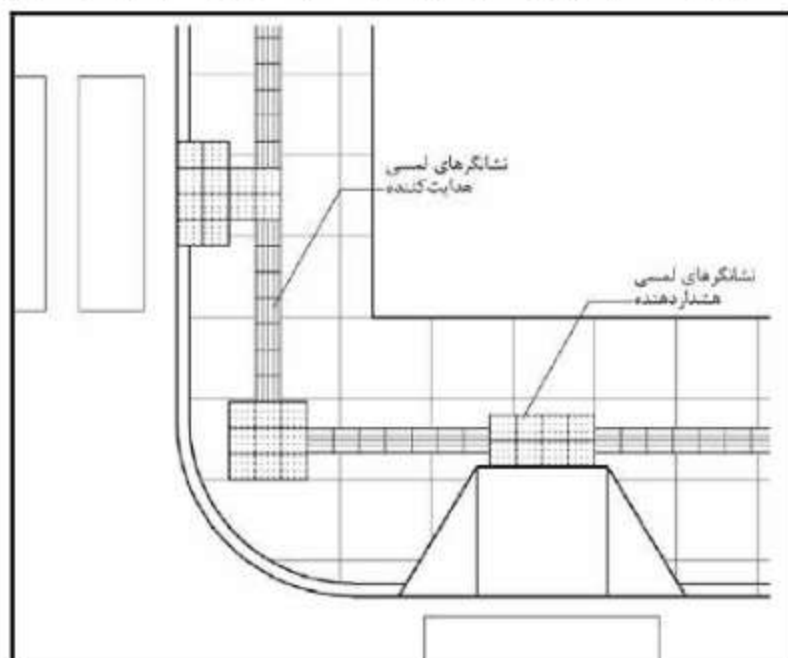
شکل ۲-۵ - نمونه کفسازی مسیر با نشانگرهای لمسی
