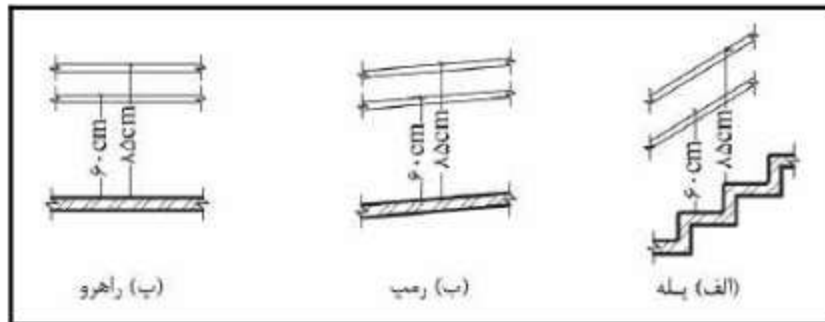
شکل ۳-۲۶- ارتفاع میله دستگرد از کف
