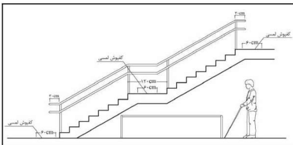
شکل ۳-۵- پاگردها در پله
