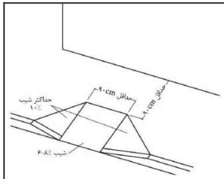
شکل ۲-۱۷- رمپ جدول
