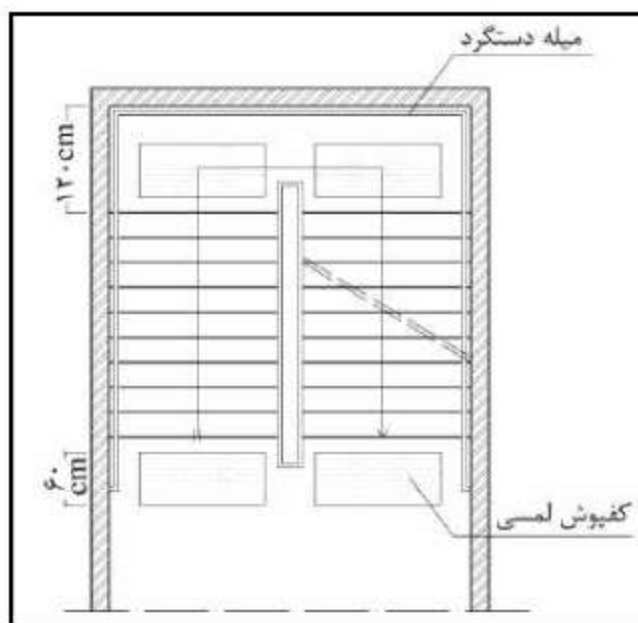
شکل ۳-۷- نصب علائم حسی در پاگرد
