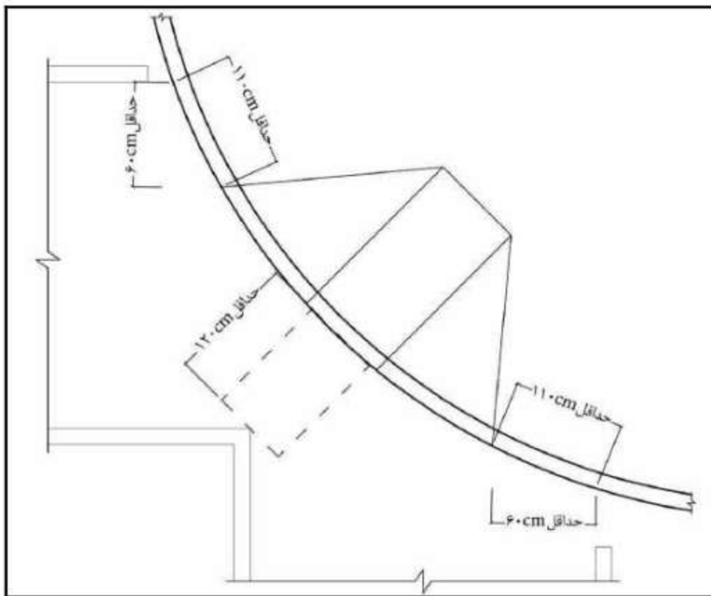
شکل ۲-۱۹- رمپ جدول قطری
