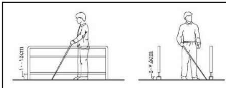
شکل ۳-۲۷- ارتفاع پایه میله دستگرد از کف
