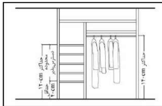
شکل ۳-۴۷- ابعاد کمد دسترس پذیر
