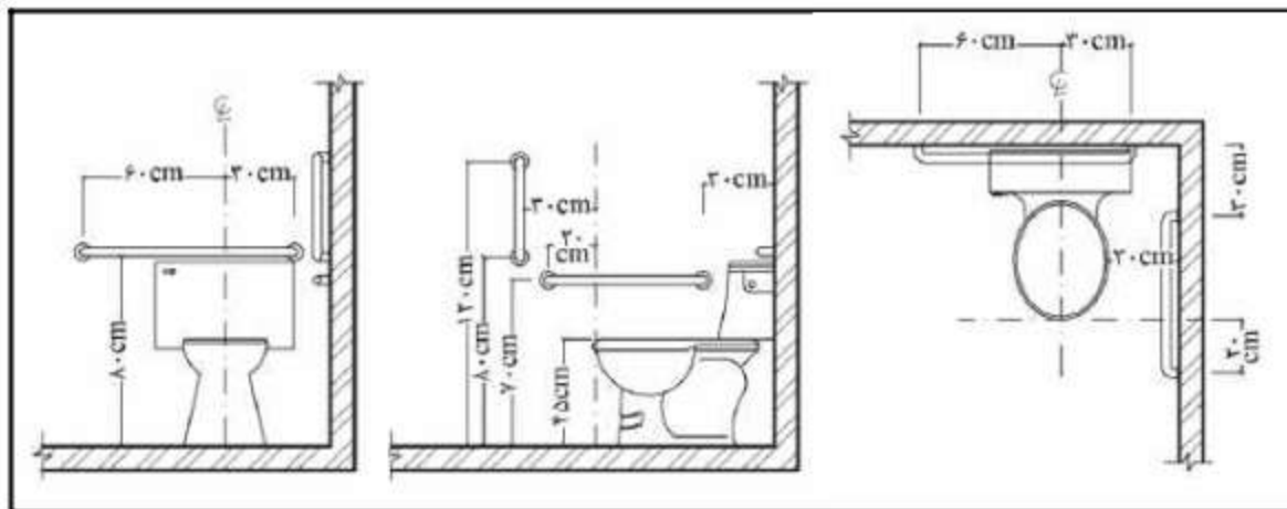
شکل ۲۹-۳- ابعاد سرویس بهداشتی فرنگی و میله دستگرد بر دیوار پشت و مجاور آن
