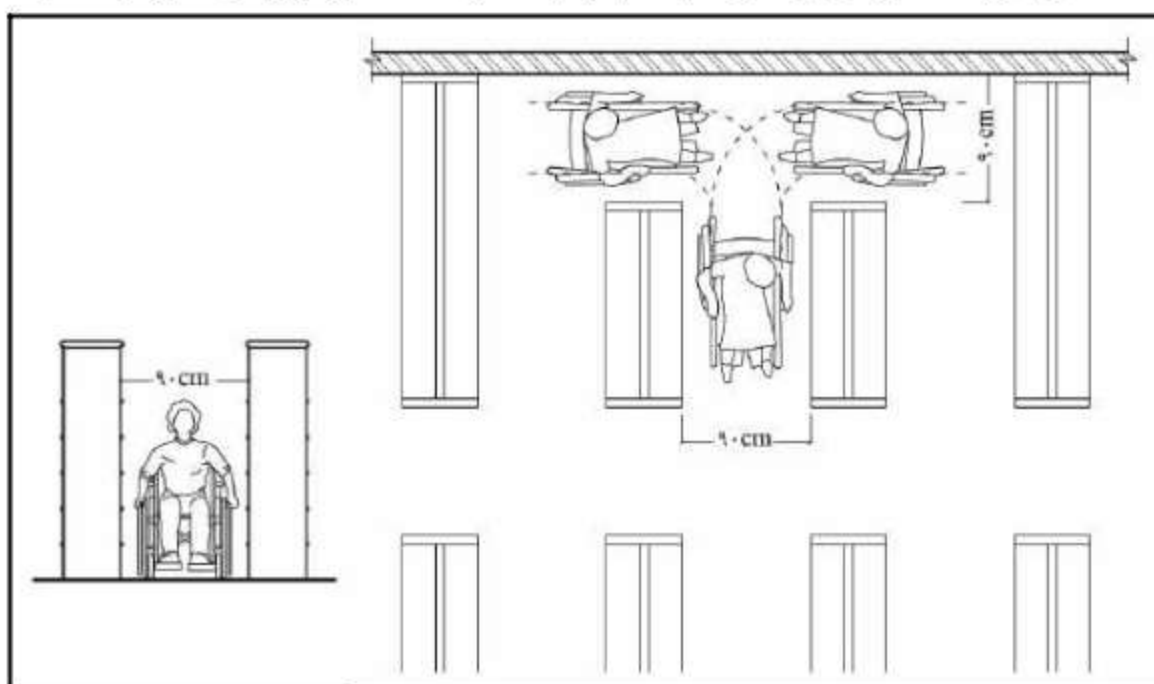
شکل ۳-۴۲- حدافل عرض آزاد مسیر بین ردیف های کتابخانه
