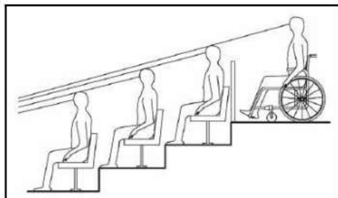
شکل ۳-۳۷- حفظ خط دید از بالای سر تماشاچیان
