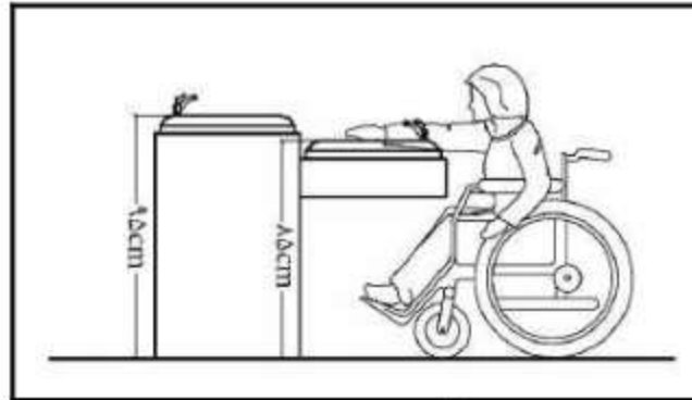
شکل ۳-۳۵- آبخوری دسترس پذیر در دو ارتفاع
