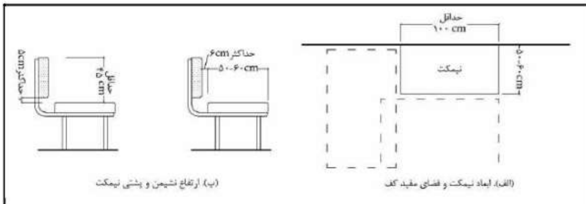
شکل ۲-۲۶ - جزئیات نیمکت در ایستگاه اتوبوس
