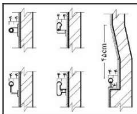
شکل ۳-۲۳- ابعاد مقطع عمودی میله دستگرد
