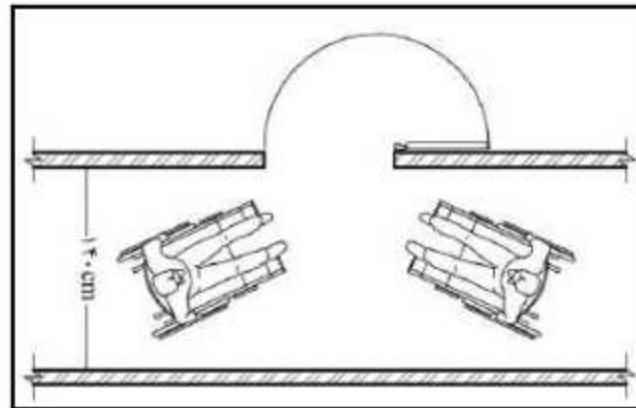
شکل ۲-۳- حداقل عرض راهرو
