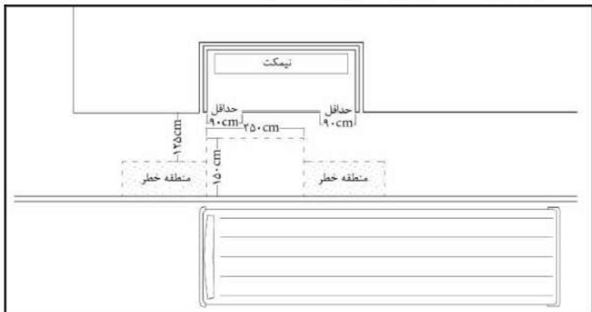
شکل ۲-۲۵- ایستگاه اتوبوس سرپوشیده
