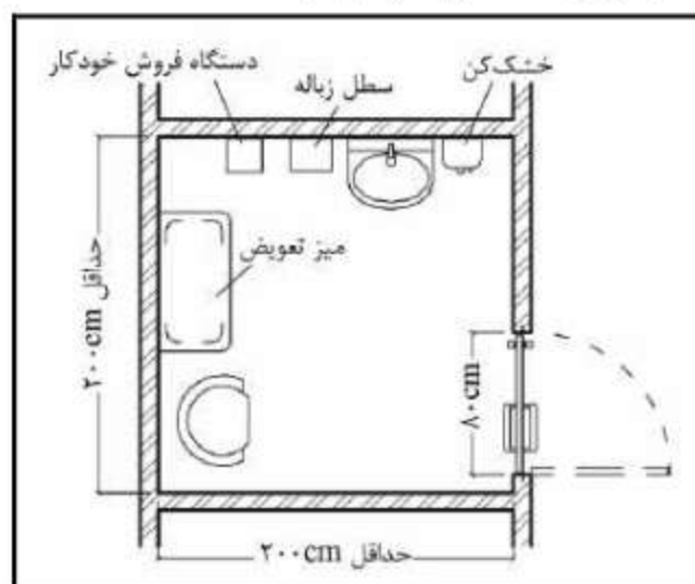
شکل ۳-۳- ابعاد و تجهیزات اتاق مادر و کودک
