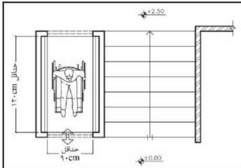
شکل ۱۵-۳- ابعاد بالابر عمودی برای طی ارتفاع ۲۰۰ تا ۴۰۰ سانتی‌متر
