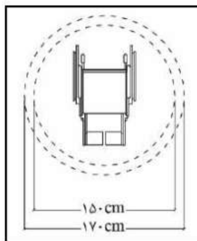
شکل ۸-۱- سطح موردنیاز برای گردش ۳۶۰ درجه‌ای صندلی چرخدار
