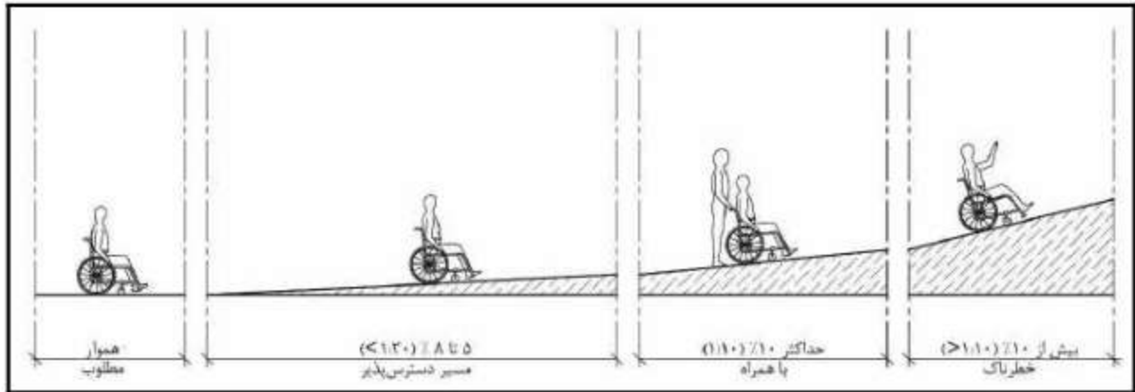
شکل ۳-۸- شیب رمپ
