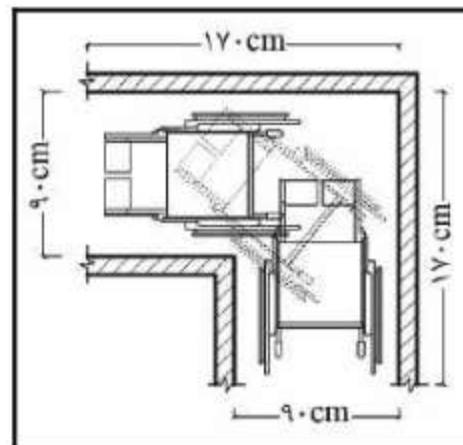
شکل ۹-۱- سطح مورد نیاز برای چرخش صندلی چرخدار از زاویه ۹۰ درجه
