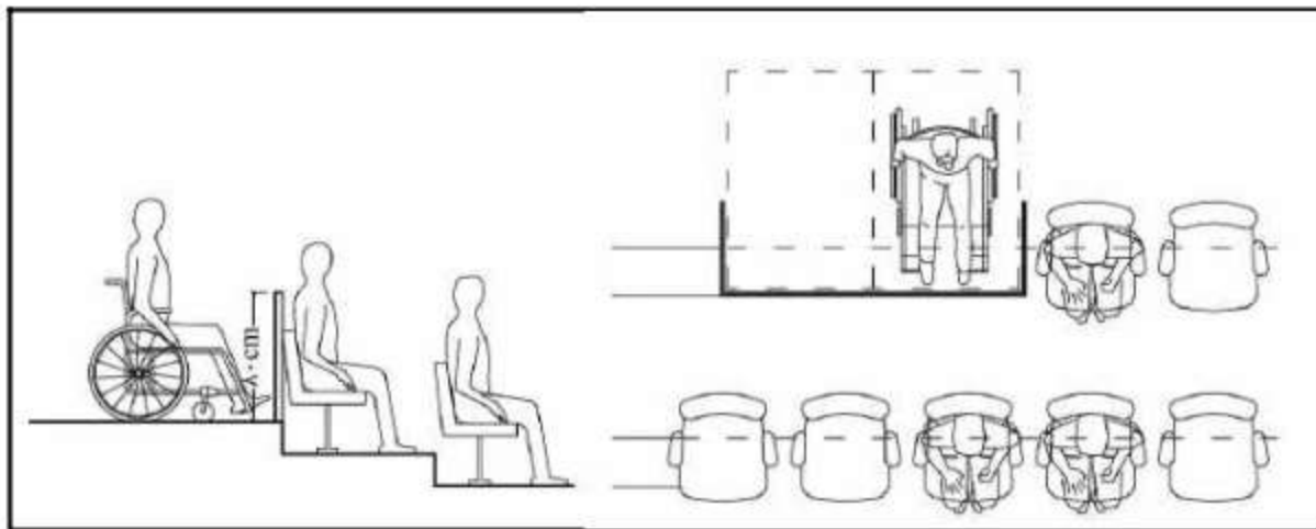
شکل ۳-۴۴- محل استقرار صندلی چرخدار در اماکن ورزشی
