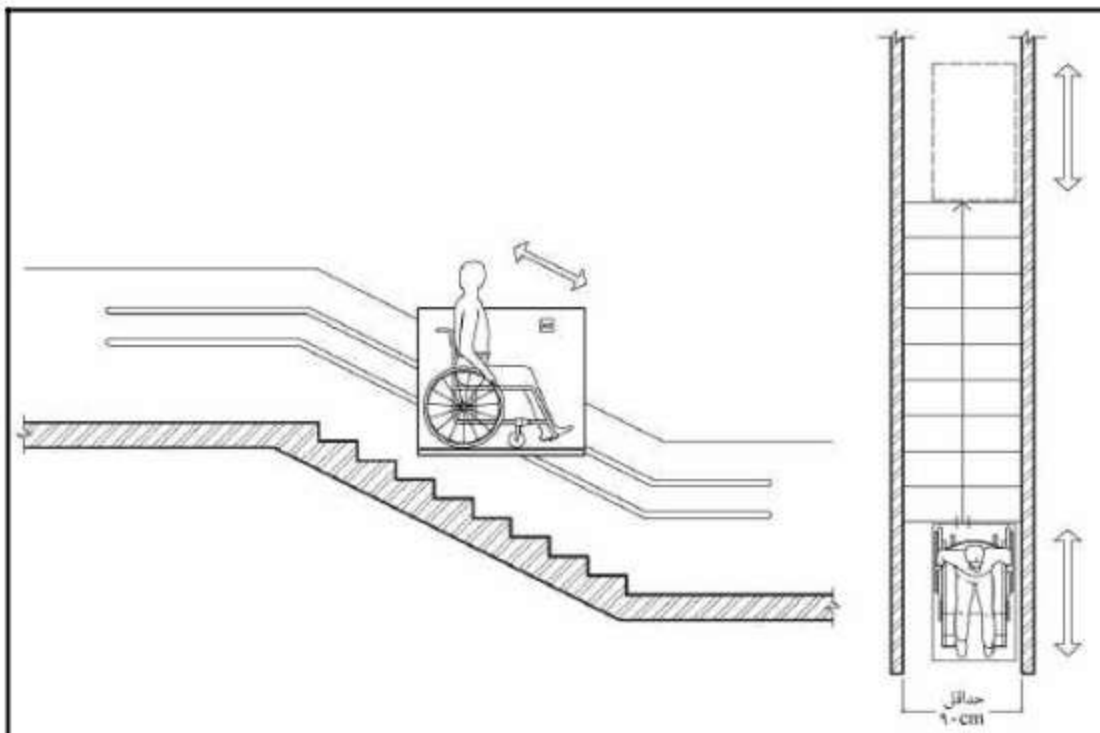
شکل ۱۶-۳- بالابر جانبی
