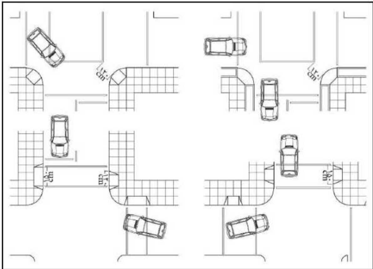
شکل ۲-۲- رمپ جدول در امتداد خط‌کشی عابر پیاده
