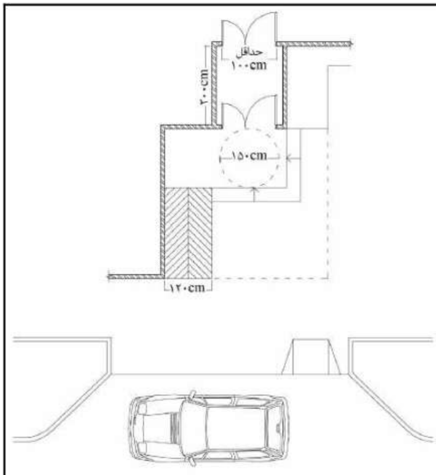
شکل ۱-۳- ابعاد و دسترسی به ورودی
