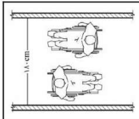
شکل ۱-۱۲- فضای مورد نیاز برای حرکت دو صندلی چرخدار بدون همراه از کنار یکدیگر
