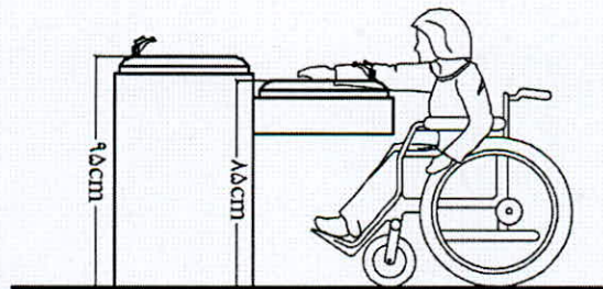
شکل شماره ۵۰: آبخوری دسترس پذیر در دو ارتفاع
