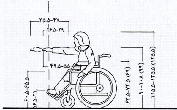
شکل شماره ۴: اندازه‌ها و دسترسی‌های زن دارای معلولیت در حرکت به جلو
