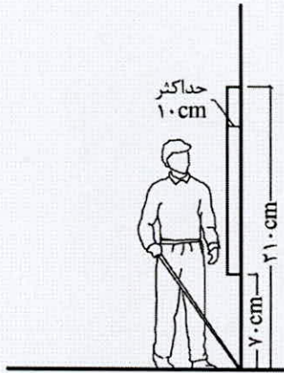
شکل شماره ۲۹: پیش‌آمدگی اشیای نصب شده روی دیوار در ارتفاع ۷۰ تا ۲۱۰ سانتیمتر
