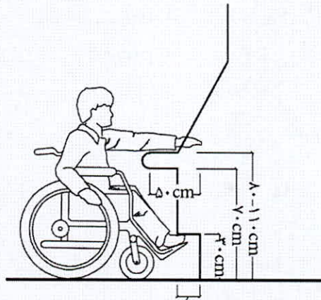
شکل شماره ۴۹: دستگاه خودپرداز دسترس پذیر
