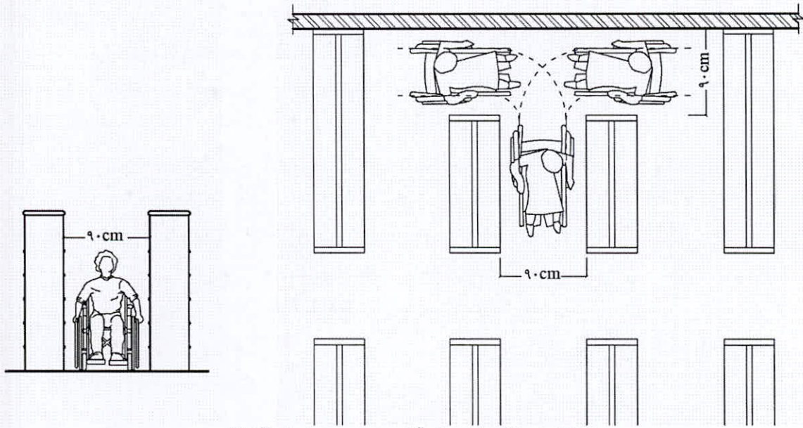
شکل شماره ۹۴: حداقل عرض آزاد مسیر بین ردیف‌های کتابخانه
