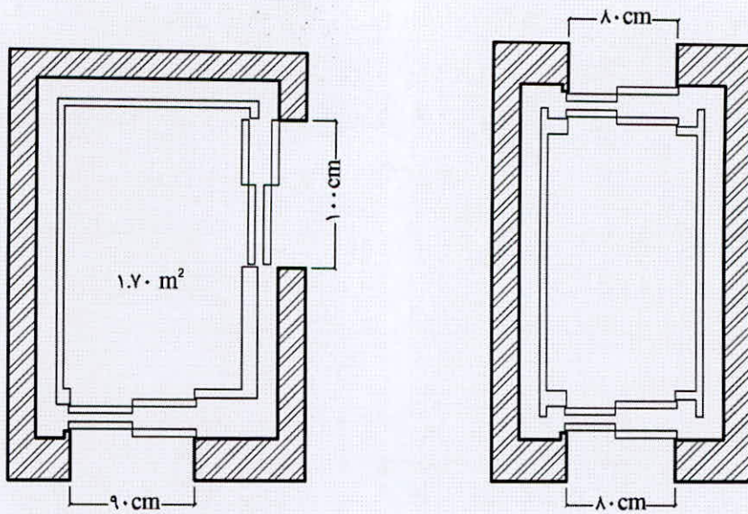
شکل شماره ۶۳: محل قرارگیری در آسانسور (الف) اتاق آسانسور با دیوارهای ۱۰۰ سانتی‌متر ارتفاع و ۹۰ سانتی‌متر عرض (ب) اتاق آسانسور با دیوارهای ۸۰ سانتی‌متر ارتفاع و ۸۰ سانتی‌متر عرض
