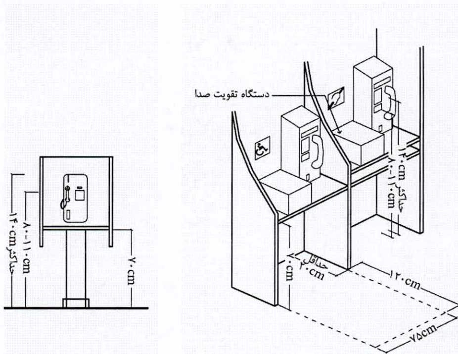
شکل شماره ۴۸: تلفن عمومی دسترس‌پذیر
