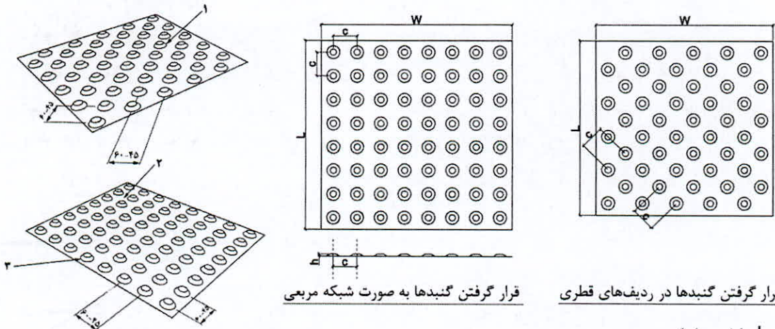
۱. قرار گرفتن مخروط‌ها در ردیف‌های قطری ۲. قرار گرفتن مخروط‌ها به صورت شبکه مربعی ۳. مخروط ناقص
