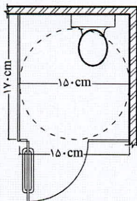
شکل شماره ۸۰: حداقل ابعاد فضای سرویس بهداشتی
