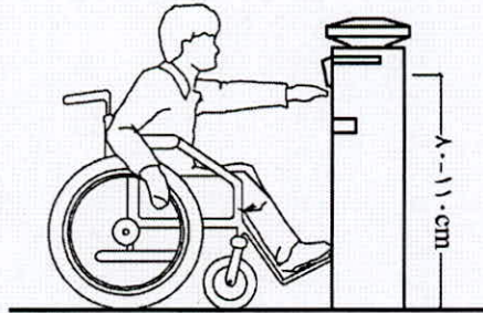
شکل شماره ۵۱: ارتفاع شکاف صندوق پست دسترس‌پذیر
