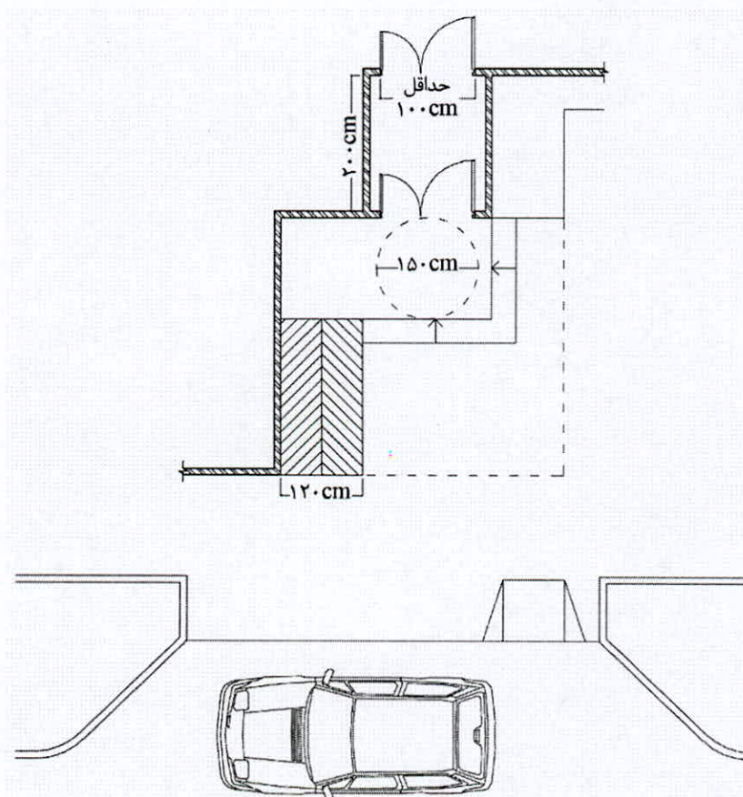
شکل شماره ۵۳: ابعاد و دسترسی به ورودی
