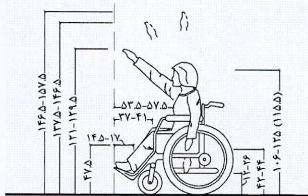
شکل شماره ۵: اندازه‌ها و دسترسی‌های زن دارای معلولیت در حرکت به بالا
